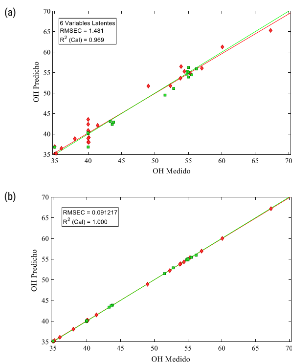
Figura 5. Curvas de calibración para la cuantificación del contenido alcohólico de muestras de Tequila Blanco mediante los modelos matemáticos (a) PLSR y (b) SVMR
