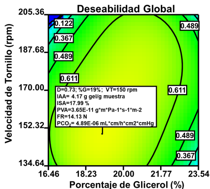
Figura 2. Gráfico de deseabilidad global ( D = 0.73 ) para obtener la combinación óptima de las variables de procesamiento (%G = 19% / VT = 150 rpm) y los valores predichos para las variables de respuesta.
