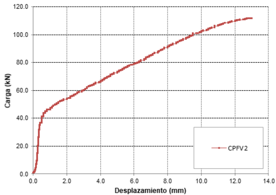
Figura 9. Curva de capacidad espécimen CPFV-2
