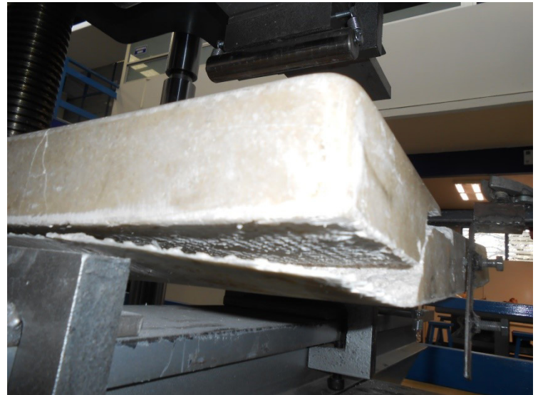
Figura 8. Desprendimiento de capa de fibra de vidrio espécimen CPFV-1
