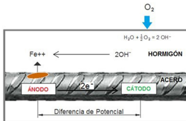
Figura 1. Proceso de corrosión en armaduras
