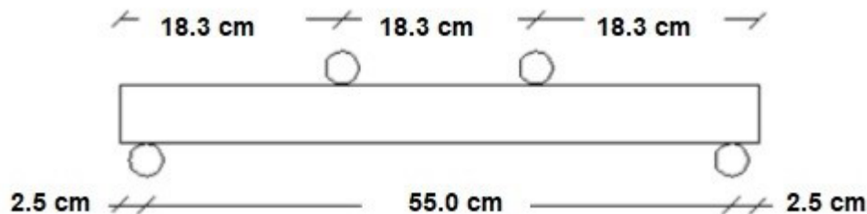
Figura 3. Condiciones de contorno del ensayo experimental
