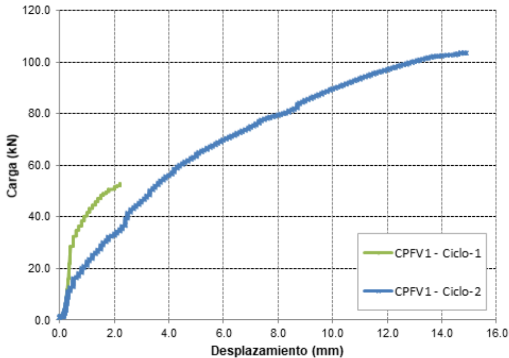
Figura 6. Curva de capacidad espécimen CPFV-1
